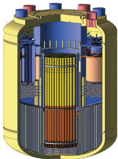
Конструкторская проработка интегрального ядерного реактора
